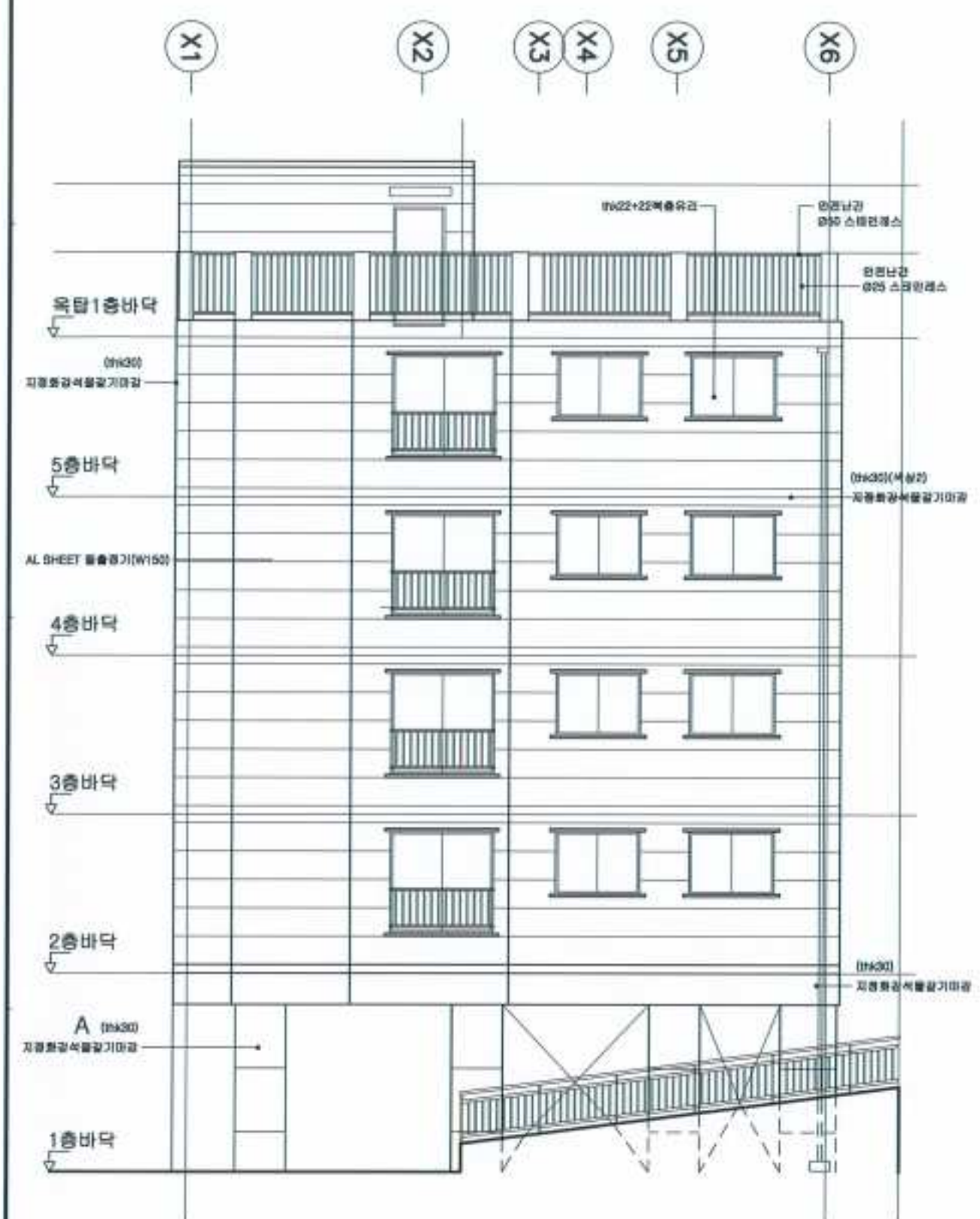
1 정면도 축척 A3 : 1/100
