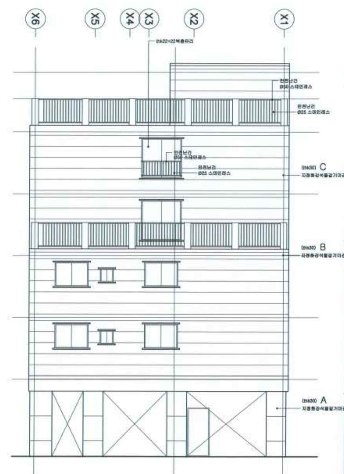
1 배면도 축척 A3 : 1/100
