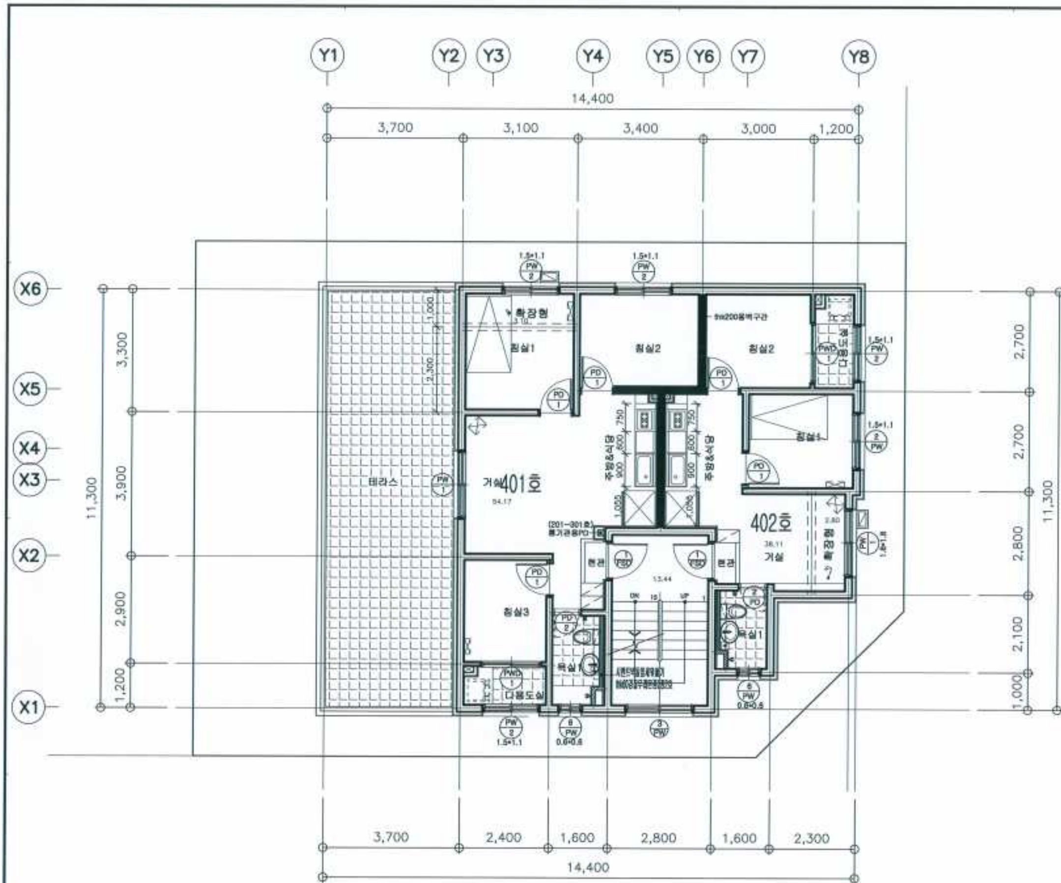
A 4층 평면도 축척 A3 : 1/100
